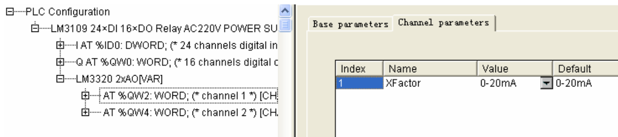
Figure 3-2-30 LM3320 Channel Parameter Configuration
